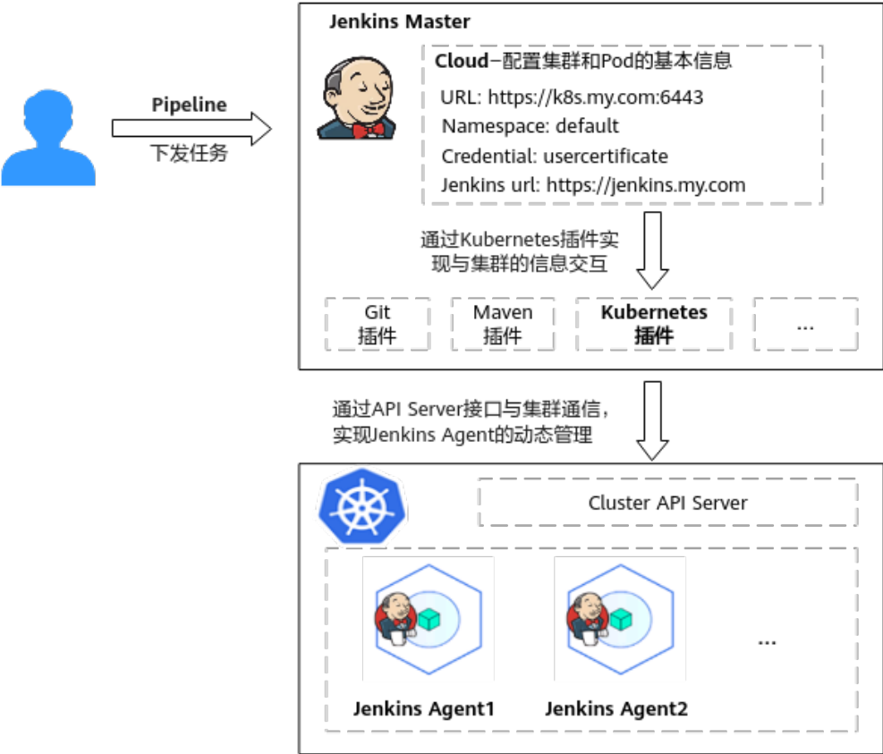
图 1-1 基本概念的逻辑关系
