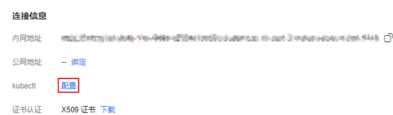
图 1-5 连接信息
