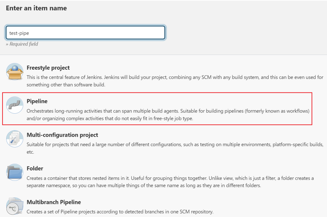
图 1-17 创建 Pipeline
