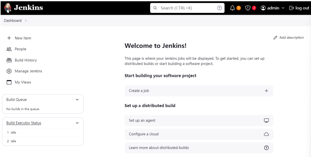
图 1-4 Jenkins 界面
